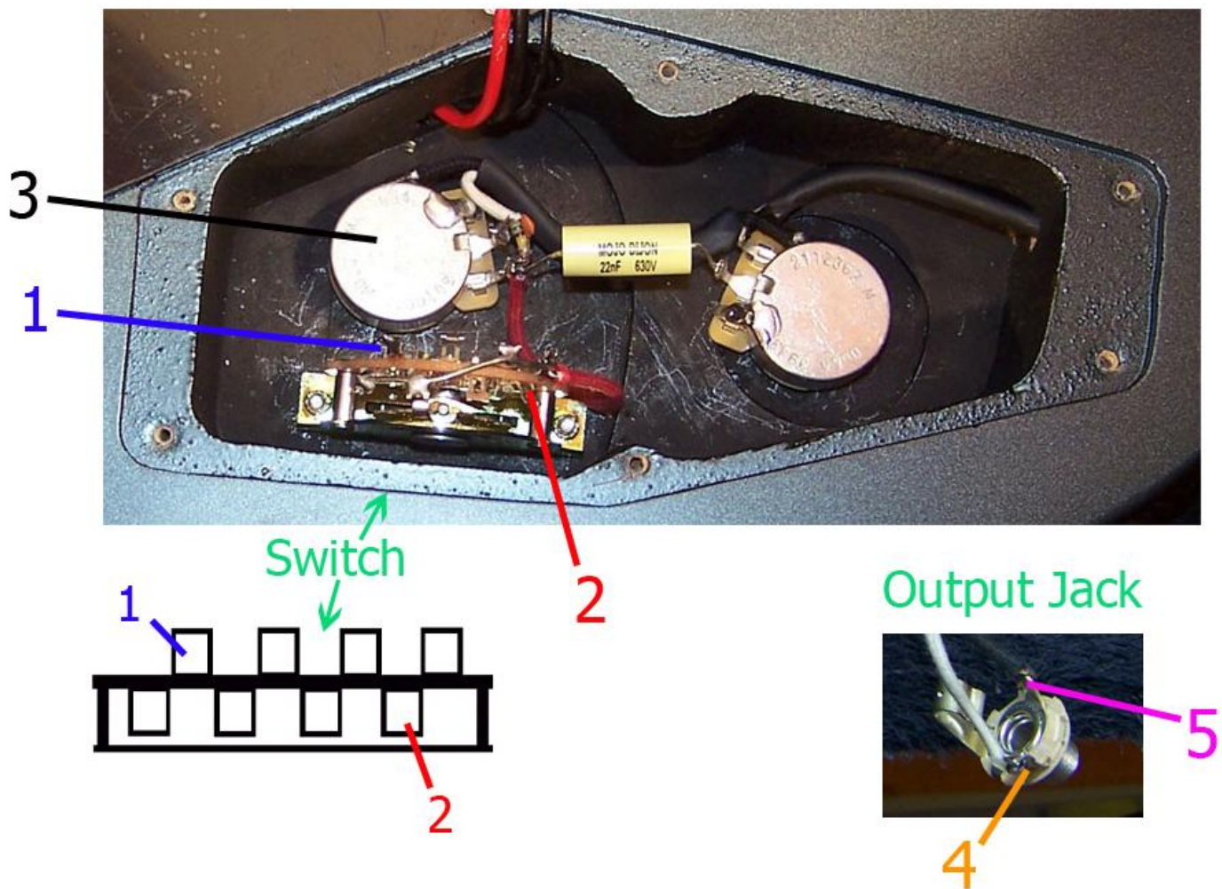
Fig. 9 Wiring layout
